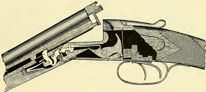
The Deeley Ejector Gun.
